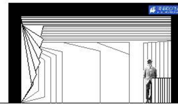
Alzado a pasillo principal, e: 1/100
